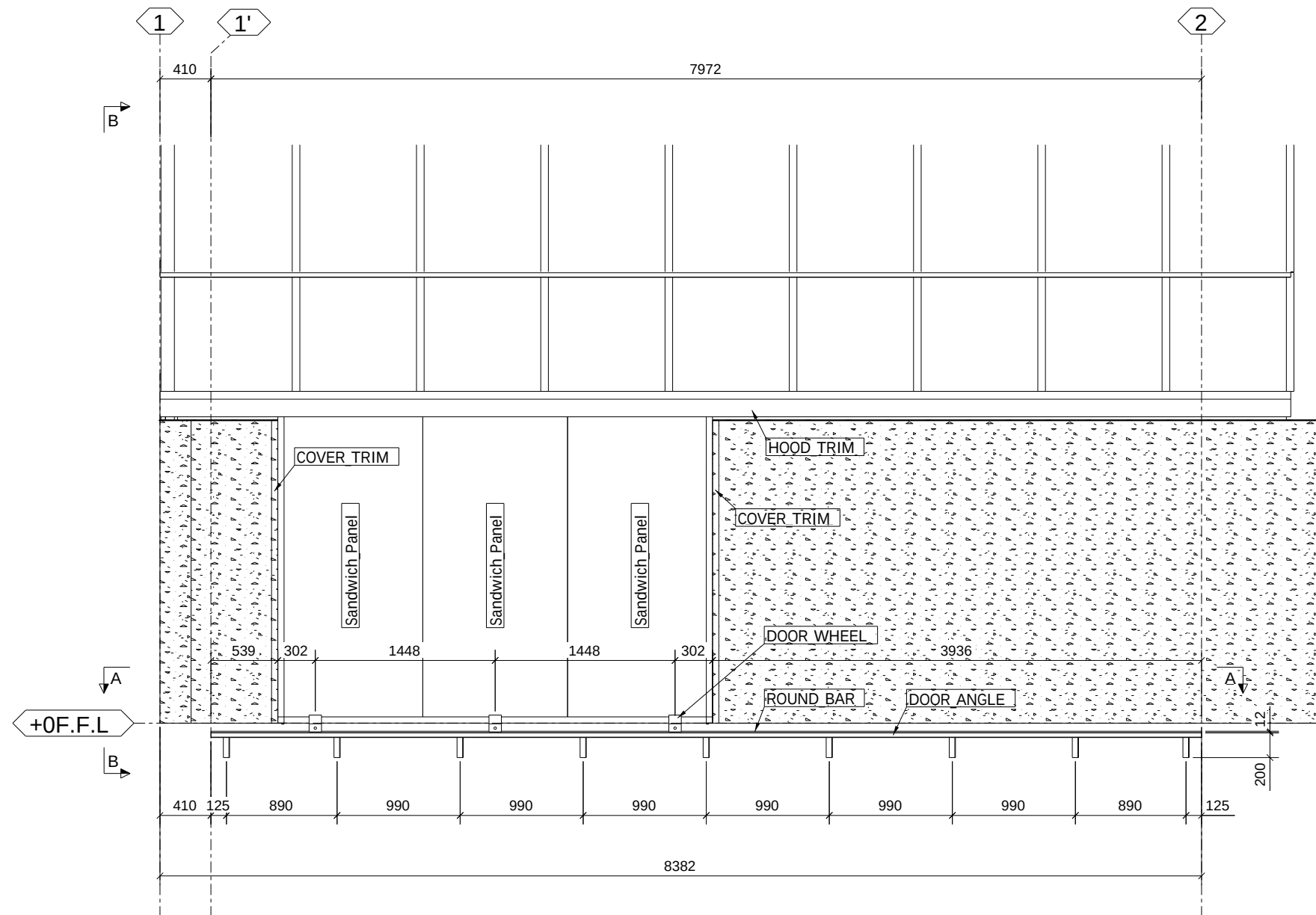
SLIDING DOOR ELEVATION
